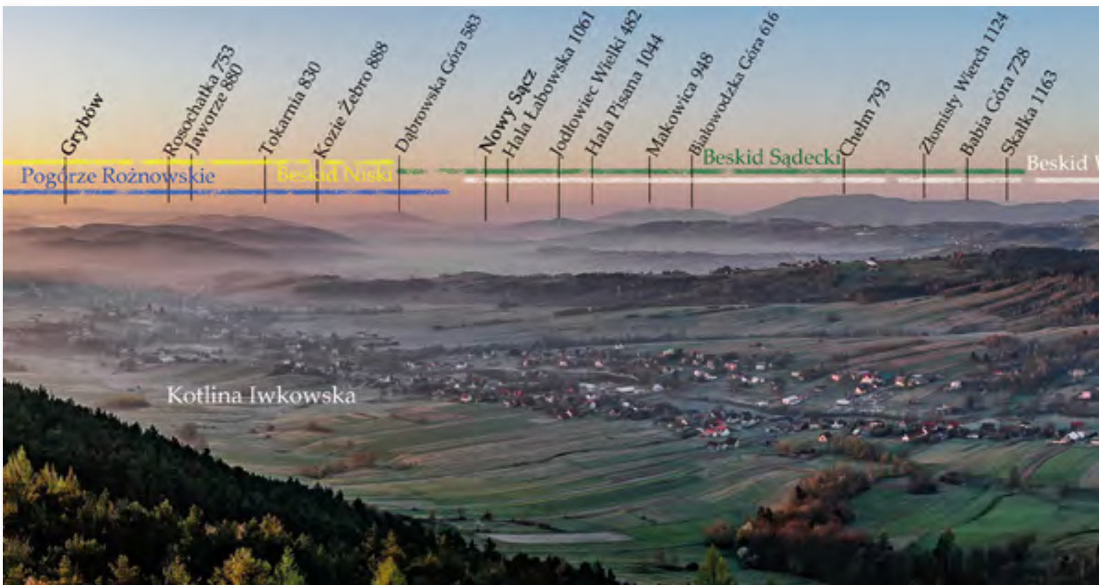
Tarnów Wal 523 Klonowa Góra 488 Bardo 534 Brzanka 534 Czychów Liwocz 562 Machulec 483 Mogiła 478 Tropie Rosulec 516 Jamna Kornuty 830 Pogórze Rożnowskie Pogórze Ciekowickie Pogórze Strzyżowskie Bukowiec 389
